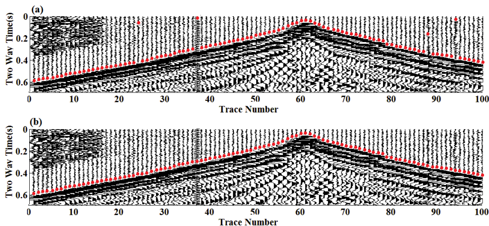
شکل ۱۶- a) نتایج مربوط به نشانگر نسبت انرژی می‌باشد که زمان اولین رسید با علامت دایره قرمز مشخص شده است. b) انتخاب‌های نادرست تصحیح شده‌اند. Fig.16. a) Results of the energy ratio attribute, where the first arrival time is marked with a red. b) Incorrect selections have been corrected.
