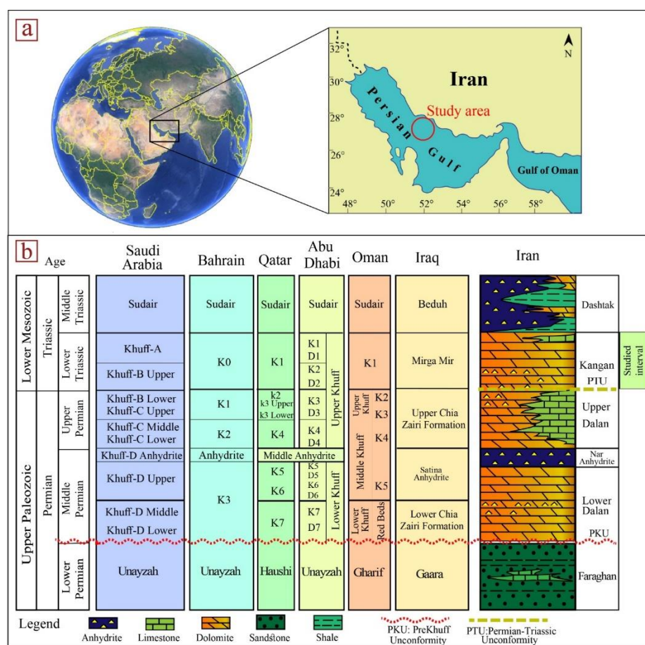
شکل ۱- a) موقعیت منطقه مورد مطالعه در بخش مرکزی خلیج فارس و b) ستون چین‌شناسی و سازند مورد مطالعه (Tavakoli and Jamalian, 2019)
