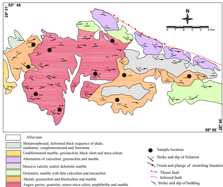
شکل ۲- نقشه زمین‌شناسی زون برشی چای کور (اقتباس از Sabzehie et al., 1996)
