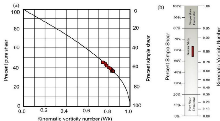
شکل ۸-ا) نمودار غیر خطی و (ب) نمودار خطی (اقتباس شده از Forte and Bailey, 2007) که رابطه بین عدد جنبش شناختی تاویی و درصد برش ساده و برش محض در جریان دو بعدی را نشان می‌دهند.
