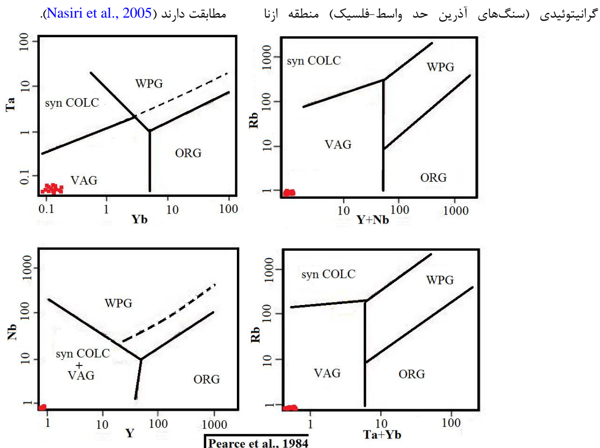
شکل ۱۰- نمودارهای تفکیک محیط‌های تکتونیکی سنگ منشأ نهشته‌های مورد مطالعه با کانی‌شناسی مشابه گرانیتوئیدها
