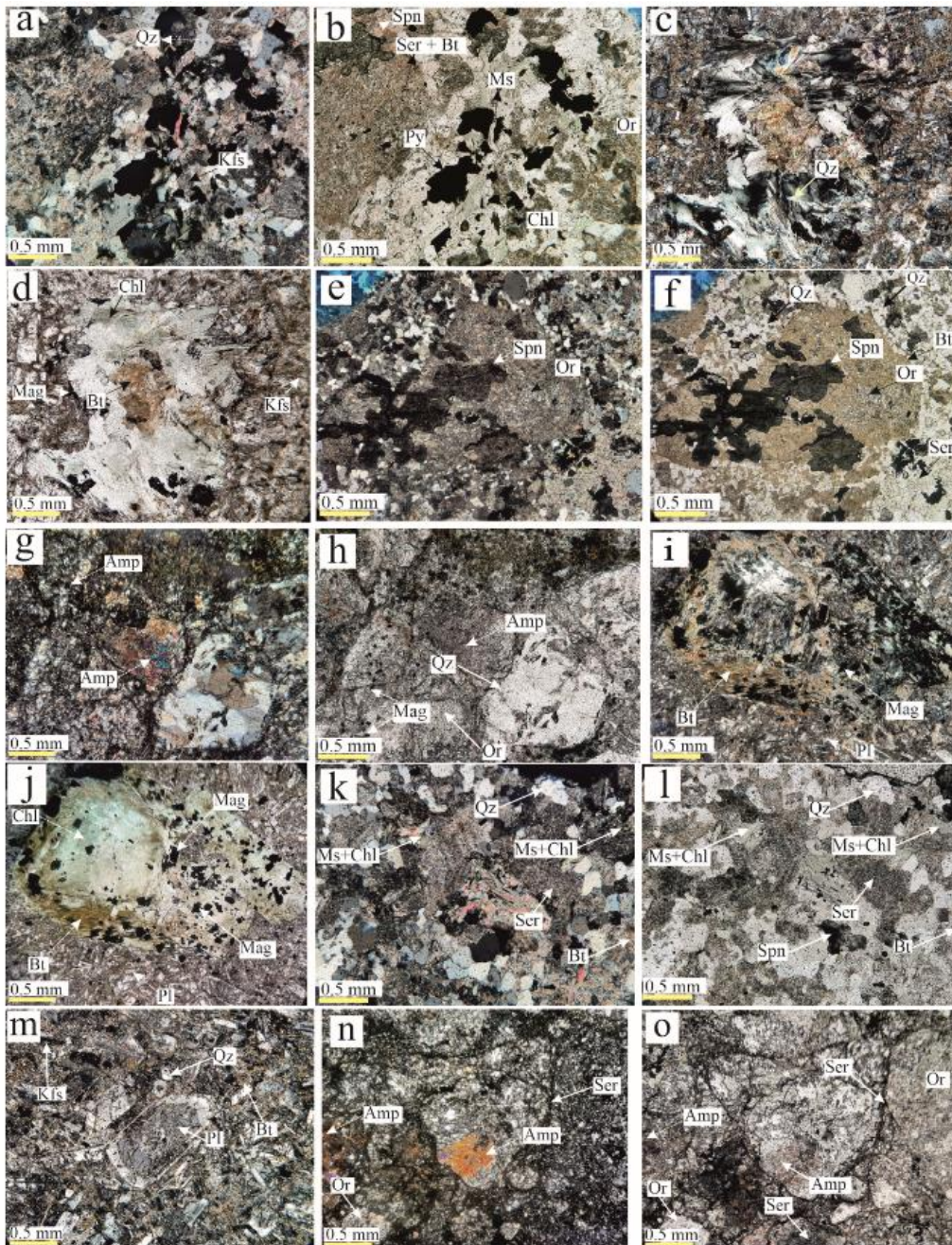
شکل ۲- تصاویر میکروسکوپی از کانی‌های سیلیکاتی گرانیت‌های کنسار میدوک: (a و b) بلورهای کوارتز با ساختار پر مانند، دگرسانی ارتوکلاز به سریسیت، دگرسانی بیوتیت به کلریت، کانی‌های فرعی و بدون شکل اسفن و پیریت و بلورهای شکل‌دار مگنتیت (شاخص زون پتاسیک در سنگ گرانیت) (a: نور XPL و b: نور PPL)، (c و d) بلورهای کوارتز با ساختار پر مانند، دگرسانی بیوتیت به کلریت، بلورهای ریز نیمه شکل‌دار مگنتیت، دگرسانی بالا فلدسپار پتاسیم به سریسیت (معرف زون پتاسیک در سنگ گرانیت) (c: نور XPL و d: نور PPL)، (e و f): بلورهای ریز بدون شکل کوارتز، بلورهای خیلی کم بیوتیت، دگرسانی ارتوکلاز به سریسیت، کانی فرعی اسفن با برجستگی تقریباً بالا (e: نور XPL و f: نور PPL)، (g و h) آمفیبول‌های دگرسان شده در یک نمونه گرانیت (g: نور XPL و h: نور PPL)، (i و j) تشکیل بیوتیت ثانویه در حاشیه کلریت در نتیجه دگرسانی گرانیت‌ها (i: نور XPL و j: نور PPL)، (k و l): دگرسانی فیلیک در گرانیت‌ها و تشکیل مسکوویت و کلریت (k: نور XPL و l: نور PPL)، (m) منطقه بندی شیمیایی در بلور پلاژیوکلاز، دگرسانی تقریباً کامل ارتوکلاز به سریسیت (معرف زون فیلیک)
