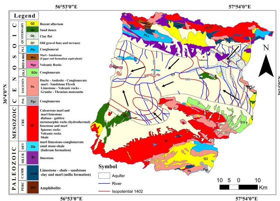
شکل ۳- نقشه هم‌پتانسیل آبخوان سبزوار (۱۴۰۲-۱۴۰۳)
