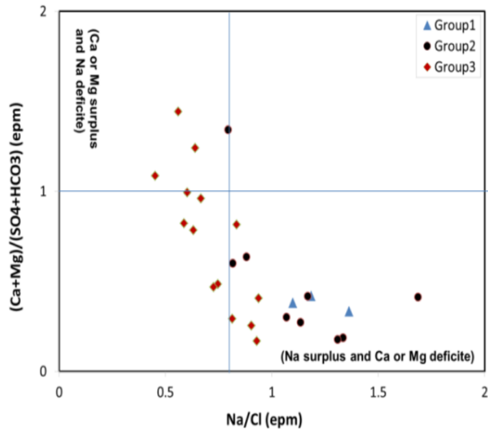
شكل ۱۳- رابطه بين \text{Ca+Mg/SO}_4\text{+HCO}_3 در مقابل نسبت \text{Na/Cl} در نمونه‌های آب‌های زیرزمینی دشت سبزوار Fig. 13. The relationship between \text{Ca+Mg/SO}_4\text{+HCO}_3 vs. \text{Na/Cl} in the water samples
