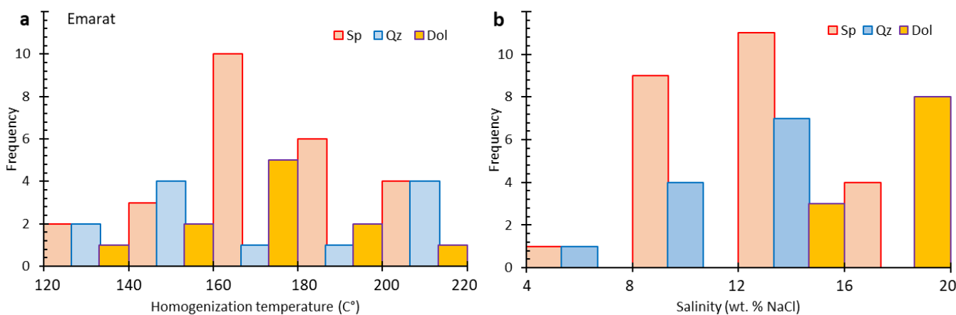
شکل ۱۰. نمودار (a) فراوانی دمای همگن‌شدگی و (b) شوری میانبرهای سیال در اسفالریت (Sp)، کوارتز (Qz) و دولومیت (Dol) از عمارت. Fig. 10. Histograms of a) homogenization temperatures and b) salinities of fluid inclusions in sphaletite (Sp), quartz (Qz), and dolomite (Dol) from Emarat.
