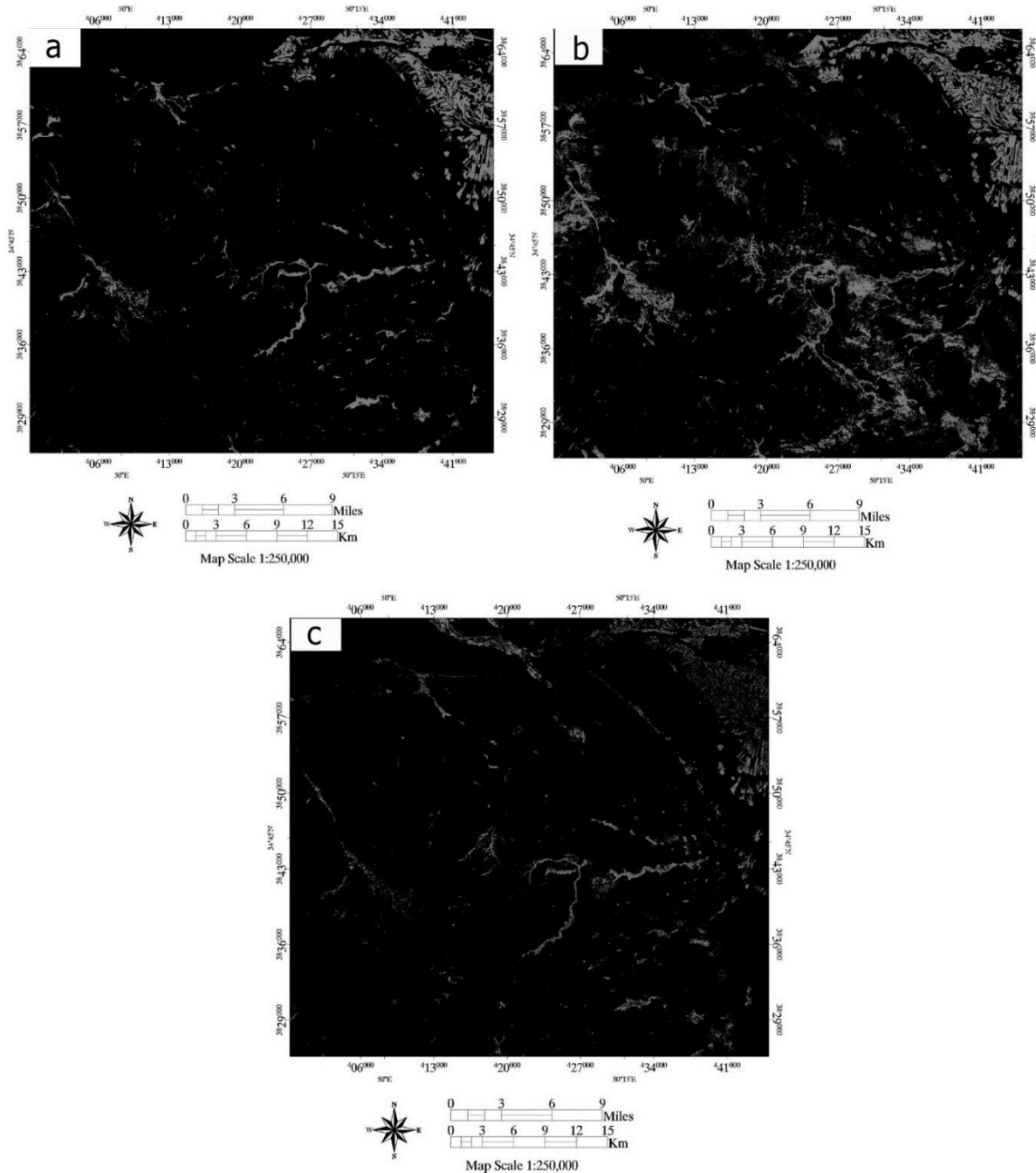
شکل ۱۷- (a) بارسازی دگرسانی آرژیلیک، (b) پروپلیتیک و (c) فیلیک به روش نقشه بردار زاویه طیفی Fig. 17. Highlighting (a) argillic, (b) propylitic, and (c) phyllic alteration using the spectral angle vector mapping method.
