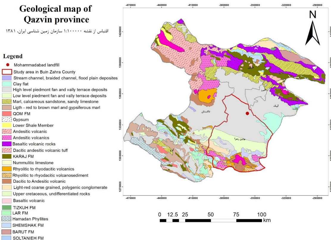
شکل ۱- نقشه زمین شناسی استان قزوین (Geological Survey of Iran, 2002) و موقعیت جغرافیایی منطقه مورد مطالعه در شهرستان بوئین زهرا Fig. 1. Geological map of Qazvin province (Geological Survey of Iran, 2002) and geographical location of the study area in Buin Zahra County
