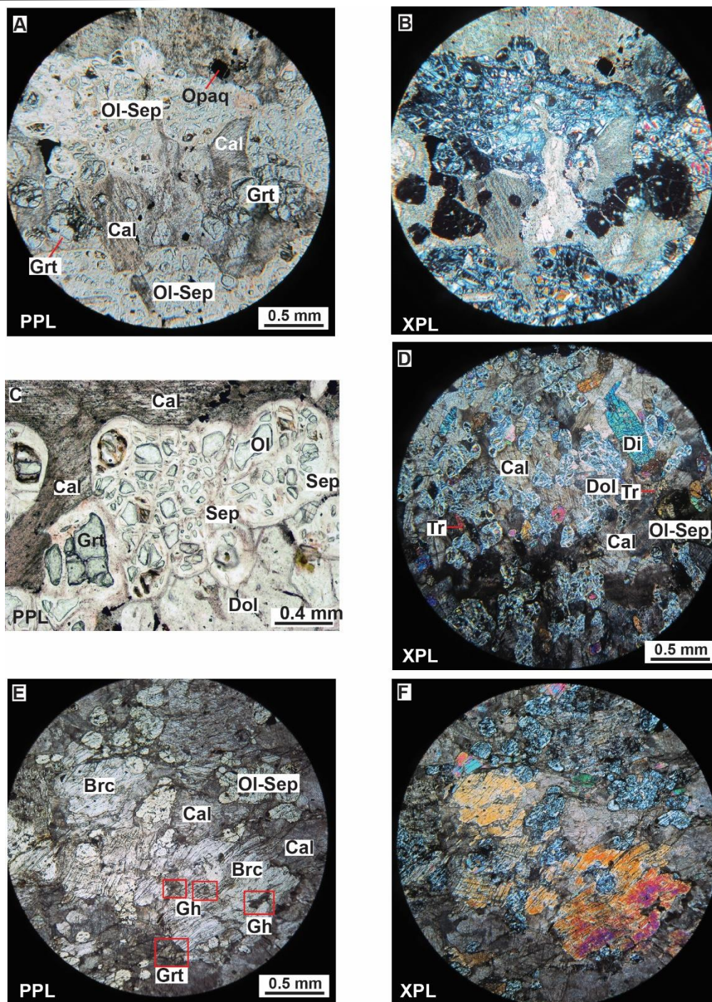
شکل ۴- تصاویر میکروسکوپی از سنگ‌های مرم دولومیتی مجموعه دگرگونی قوری. (a و b) رخداد گردهمایی کانیایی الیوین + گارنت + دیوپسید + کلسیت + دولومیت در سنگ‌های با درجه دگرگونی قوی در طول دگرگونی M1 به سمت M2 که در مراحل بعدی دگرگونی (انتهای M2)، الیوین به سرپانتین (آنتی‌گوریت) و گارنت به سریسیت و کلریت (پینییتی شدن) تبدیل شده‌اند. (c و d) رخداد گردهمایی کانیایی الیوین + دیوپسید + کلسیت + دولومیت + کانی کدر در سنگ‌های با درجه دگرگونی قوی در طول دگرگونی M2 (به شکل ۶ مراجعه شود). الیوین‌ها در مراحل بعدی دگرگونی الیوین، سرپانتینی (آنتی‌گوریت) شده‌اند و بلورهای
