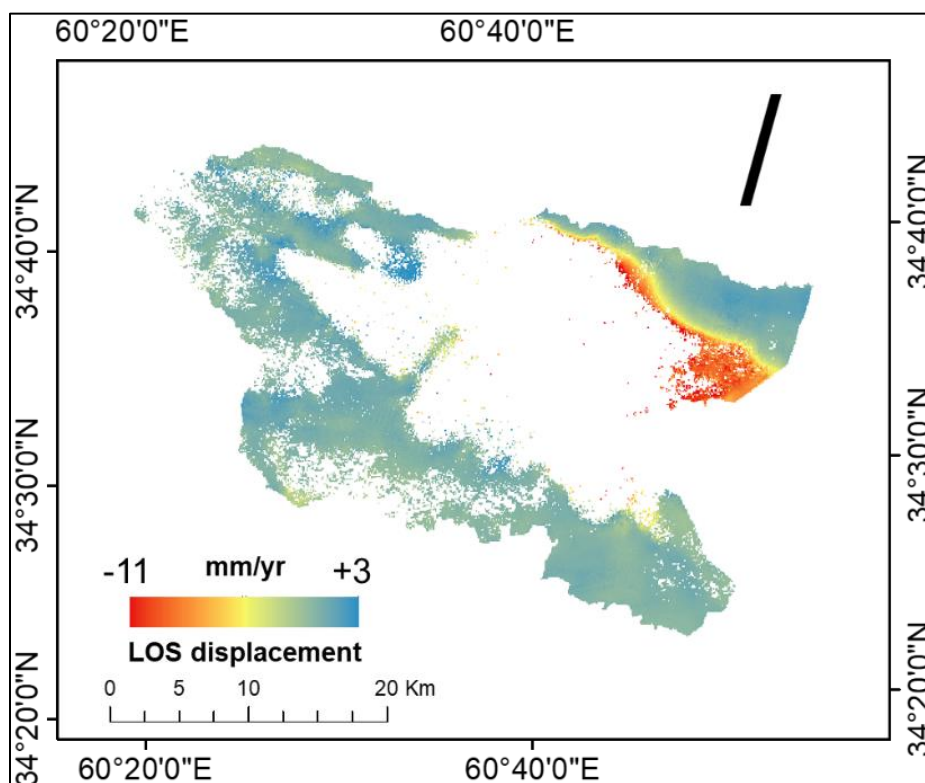
شکل ۱۲- مقادیر فرونشست دشت کرات حاصل از تصاویر ماهواره‌ای (ASAR) (1385-1398)
