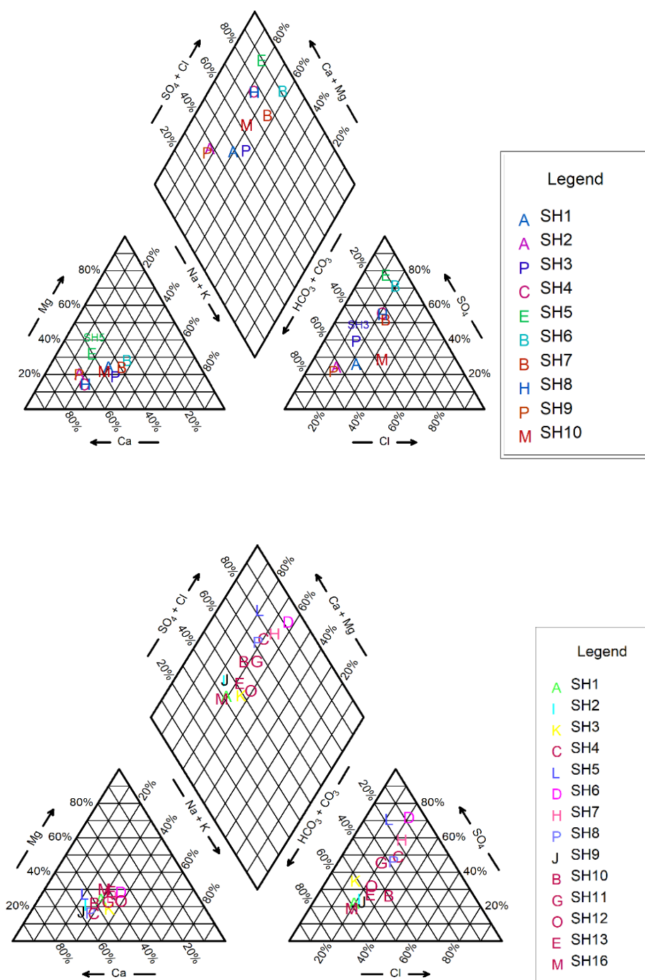
شکل ۸- نمودار پایپر نمونه‌های آب‌بازرسی آبخوان شوش در دوره‌های سیلابی (بالا) و خشک (پایین) Fig. 8. Piper diagram of the Shush groundwater in flood (above) and dry (below) period
