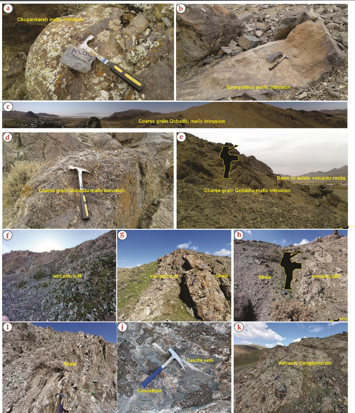
شکل ۳- a, b, c) نمای از رخنمون توده‌های گابرویی قبادلو، چوپانکره و قره‌قشون. d) رخنمون گابروی قبادلو و واحدهای اسیدی و بازیک. e, f, g) کنتاکت واحدهای توفی و شیلی با واحدهای گابرویی. h, i, j) واحدهای شیلی و آهکی. k) واحدهای کنگلومرایی.
