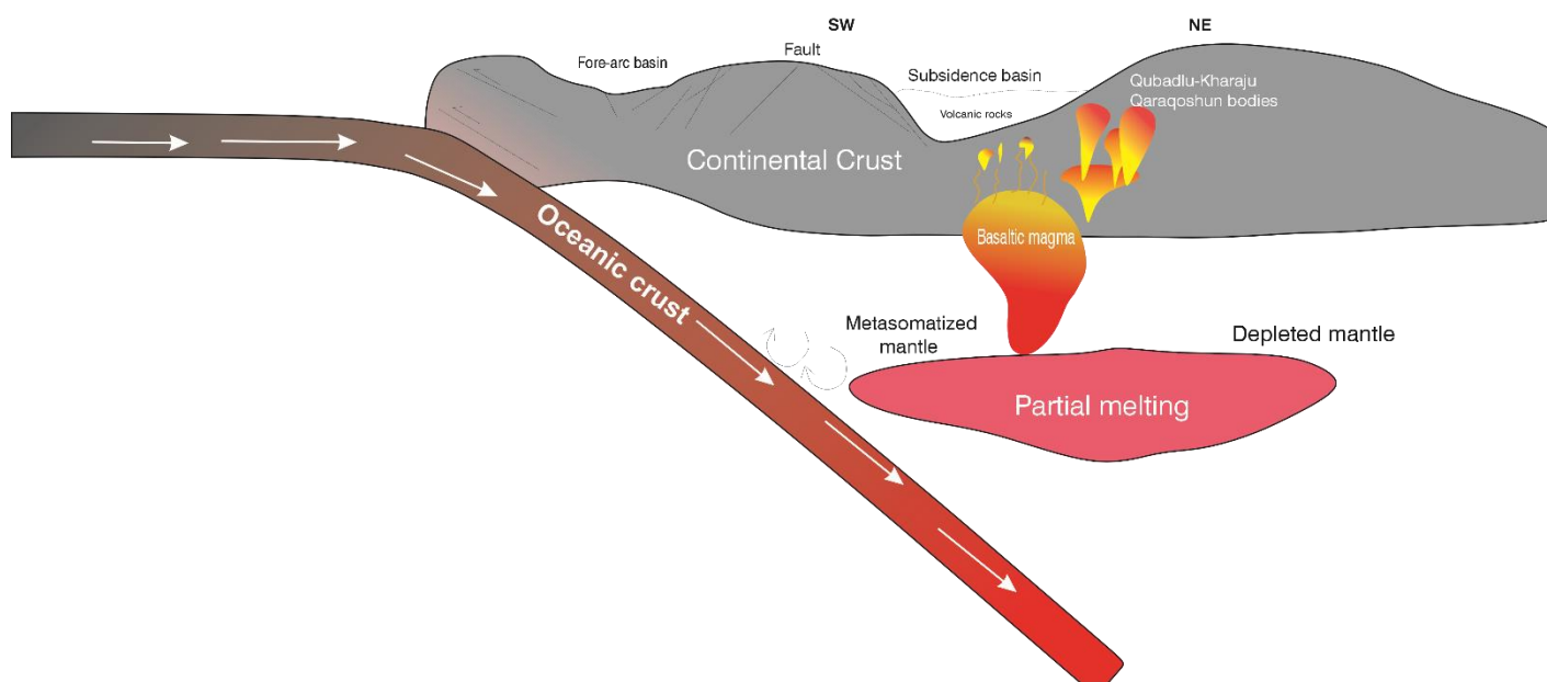
شکل ۱۳- تصویری شماتیک از مدل بخش شمالی زون سنندج-سیرجان و ماگماتیسم کرتاسه در این زون.
