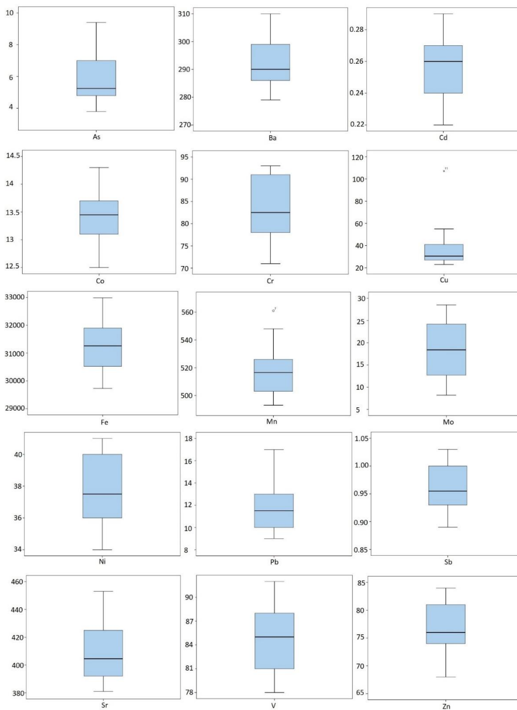
شکل ۴- نمودار جعبه‌ای غلظت عناصر (بر حسب mg/kg) در خاک‌های کشاورزی دشت بسطام (سال ۱۴۰۲) Fig. 4. The box plots of elements concentration (in mg/kg) in the agricultural soils of the Bastam Plain (2023)
