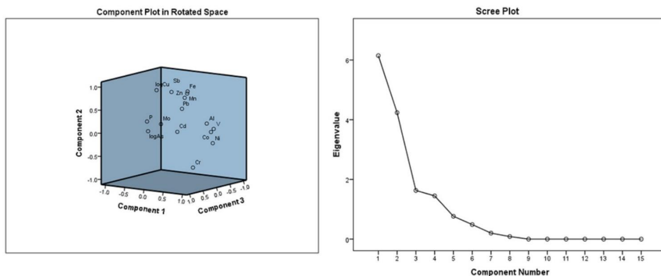
شکل ۸- نمودار صخره‌ای و نمودار بارگذاری مؤلفه‌ها برای عناصر مورد مطالعه در خاک کشاورزی دشت بسطام Fig. 8. The scree plot and loading diagram of components for the studied elements in the agricultural soils of the Bastam Plain
