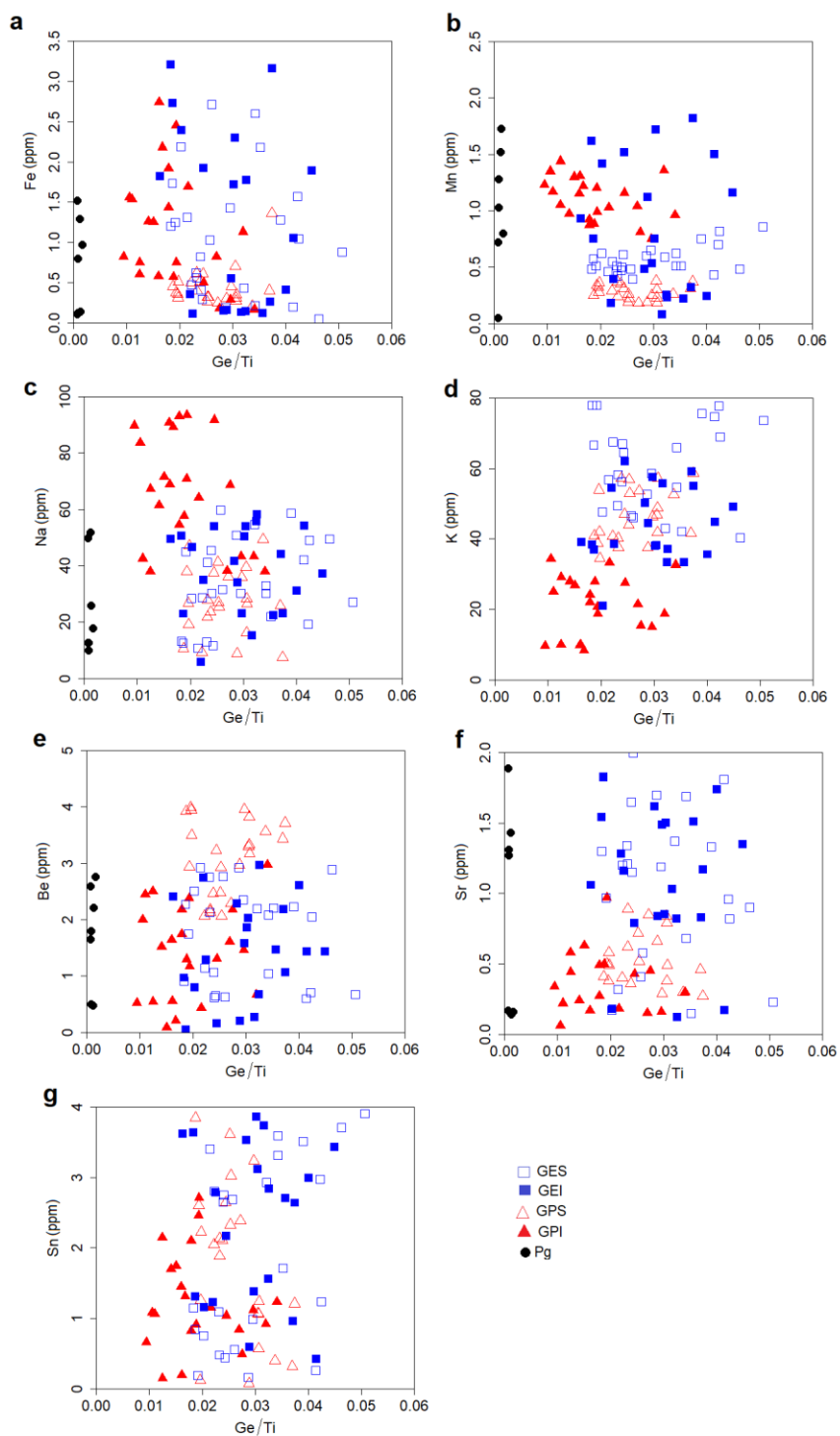
شکل ۷- نمودارهای دوتایی Ge/Ti در مقابل عناصر کیمیایی که توزیع نامنظم در بلورهای کوارتز دارند. علائم همانند شکل ۵ هستند.
