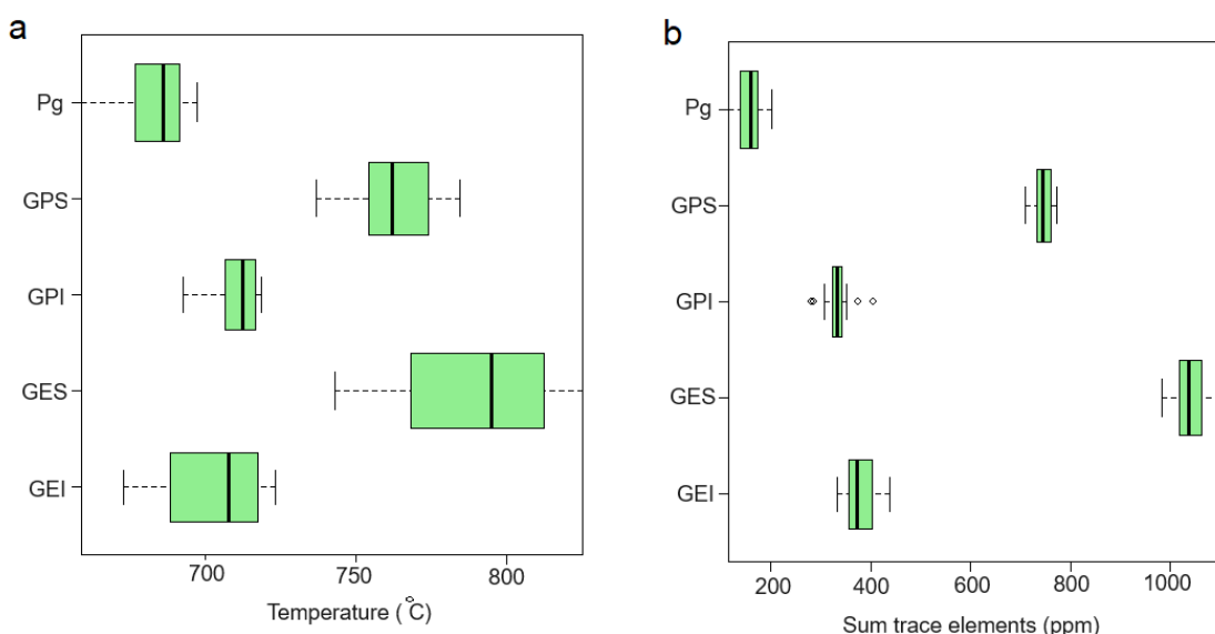
شکل ۸- a) مقایسه دمای محاسبه شده با روش Titan Q بلورهای کوارتز در انواع گرانیتوئیدهای مورد مطالعه. b) تفاوت مجموع عناصر کیمیا در انواع گرانیتوئیدها. : گرانیتوئیدهای نوع S در منطقه کبودان؛ GPI: گرانیتوئیدهای نوع I در منطقه کبودان؛ GES: گرانیتوئیدهای نوع S در مجموعه نفوذی بانه؛ GEI: گرانیتوئیدهای نوع I در مجموعه نفوذی بانه؛ Pg: پلاژیوگرانیت‌های سبزوار.
