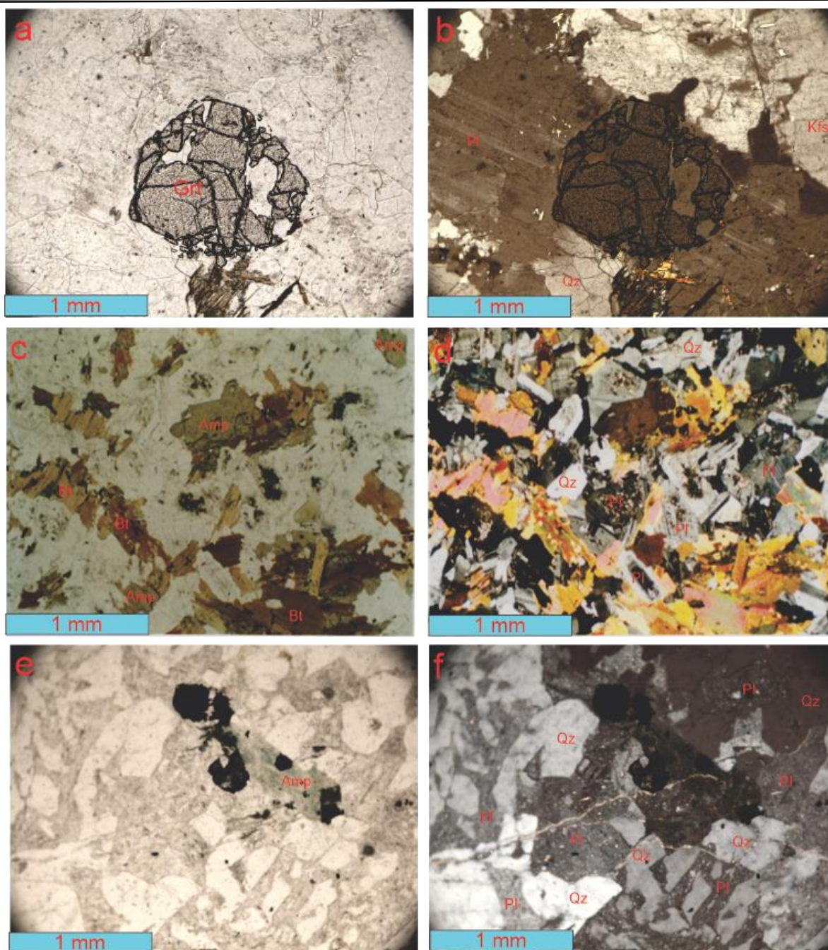
شکل ۴- خصوصيات بافتي گرانيت نوع S از مجموعه نفوذی بانه در نور پلاریزه ساده (a) و نور پلاریزه متقاطع (b). یک نمونه از گرانودیوریت نوع I از همین مجموعه در نور پلاریزه ساده (c) و پلاریزه متقاطع (d). نمایی از بافت یک پلاژیوگرانیت در مجموعه افیولیتی شمال سبزوار با هم رشدی گرافیکی کوارتز و پلاژیوکلاز در نور پلاریزه ساده (e) و متقاطع (f). Amp: آمفیبول، Bt: بیوتیت، Grt: گارنت، Kfs: فلدسپار پتاسیم، Pl: پلاژیوکلاز.
