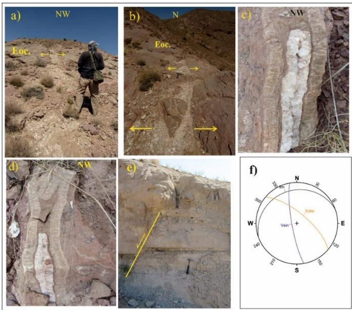
شکل ۶- a و b) شکستگی‌های کششی سیلیسی در پلتفرم کربناته شمال بیرجند. c و d) رگه‌های کششی syntaxial در منطقه چاه‌حوض. e) گسلش نرمال در آهک و مارن‌های شمال بیرجند. f) استریوگرام توزیع دایک‌ها و شکستگی‌های کششی در محدوده نیم‌رخ صحرائی B در شکل ۲.
