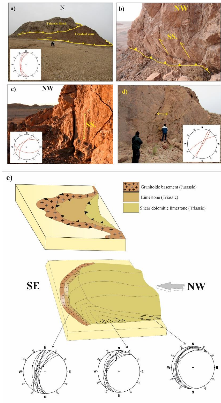
شکل ۴-ا) راندگی آهک تریاس (Tri.) و پهنه خرد شده گسلی در منطقه سه‌چنگی (محدوده Th.2 در شکل ۲). ب) راندگی جانبی با خش‌لغزهای مایل و شیب صفحه گسل به سمت شمال غرب. ج) نمای از جبهه راندگی با خش‌لغزهای قائم و استریوگرام آن. د) خش‌لغزهای نیمه افقی در بخش جانبی راندگی. تصویر شماتیک از پهنه راندگی و وضعیت خش‌لغزهای موجود در بخش پیشانی (جبهه) و جانبی برگه‌های راندگی به همراه استریوگرام‌های مربوطه. علامت پیکان: جهت انتقال زمین‌ساختی در منطقه.
