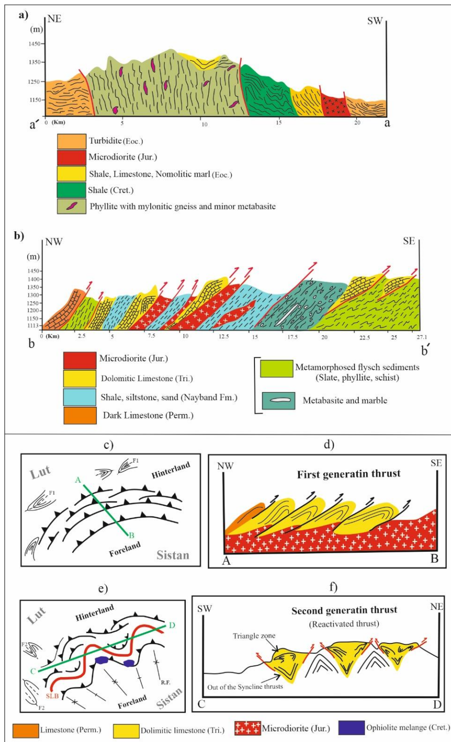
شکل ۱۰ - a و b) نیمرخ‌های عرضی ترسیم شده از منطقه سه‌چنگی. موقعیت نیمرخ‌ها در شکل ۱۰ نشان داده شده است. c تا f) مدل تکامل تکتونیکی منطقه سه‌چنگی در مرز خمیده شمالی پهنه‌های ساختاری لوت-سیستان که عبارتند از: c) هندسه راندگی‌ها و چین‌های موازی نسل اول از حادثه دگرشکلی اول در زمان پالئوسن میانی. d) مقطع عرضی از شکل c که خصوصیات برگه‌های راندگی نسل اول
