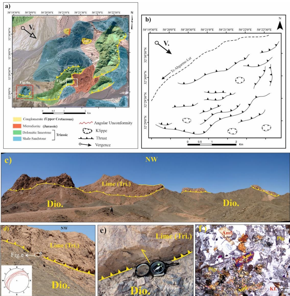
شکل ۳- a) ارتباط بین واحدهای زمین‌شناسی مختلف با صفحات راندگی در منطقه سه‌چنگی. V.: جهت انتقال زمین‌ساختی. (b) نقشه ساختاری از راندگی‌های شکل a. (c) تصویر پانوراما از راندگی آهک‌های تریاس (Tri.) بر روی میکرودیوریت‌های ژوراسیک (Dio.). (d) کنتاکت گسلش راندگی بین آهک و میکرودیوریت. کادر روی تصویر در شکل e بزرگنمایی شده است. (e) صفحه گسلش راندگی با شیب به سمت شمال غرب. (f) مقطع نازک میکروسکوپی از میکرودیوریت منطقه سه‌چنگی. بافت میکروگرانولار شامل کانی‌های فلدسپار (Kf)، پلاژیوکلاز (Plg.) و آمفیبول (Amf.). نورپلاریزه با بزرگنمایی ۴۰ برابر.
