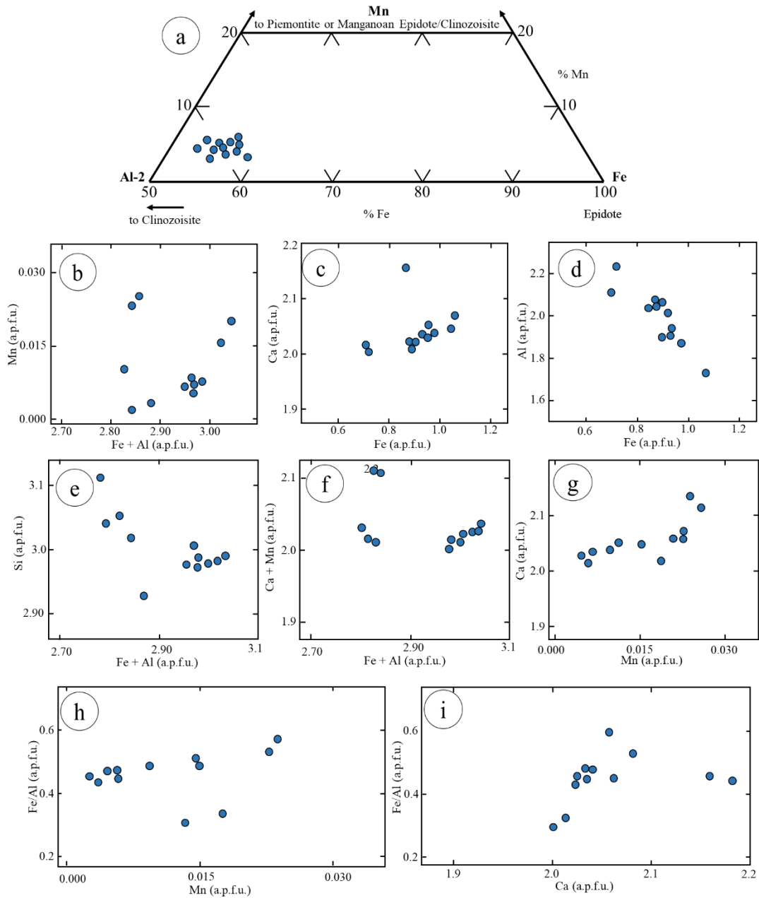
شکل ۲۱- داده‌های کانی اپیدوت حاصل از تجزیه EPMA. (a) طبقه‌بندی به عنوان اپیدوت واقعی. (b-i) روابط بین کاتیون‌های اصلی واقع در ساختار اپیدوت. (توجه داشته باشید که تمام داده‌های نشان داده شده در pfu بر اساس ۲۵ اتم اکسیژن محاسبه شده‌اند). Fig. 21. EPMA data of epidote. a) Classification of epidotes, b-i) Relationships between major cations in the epidote structure. (Note that all the data shown in pfu are calculated based on 25 oxygen atoms).
