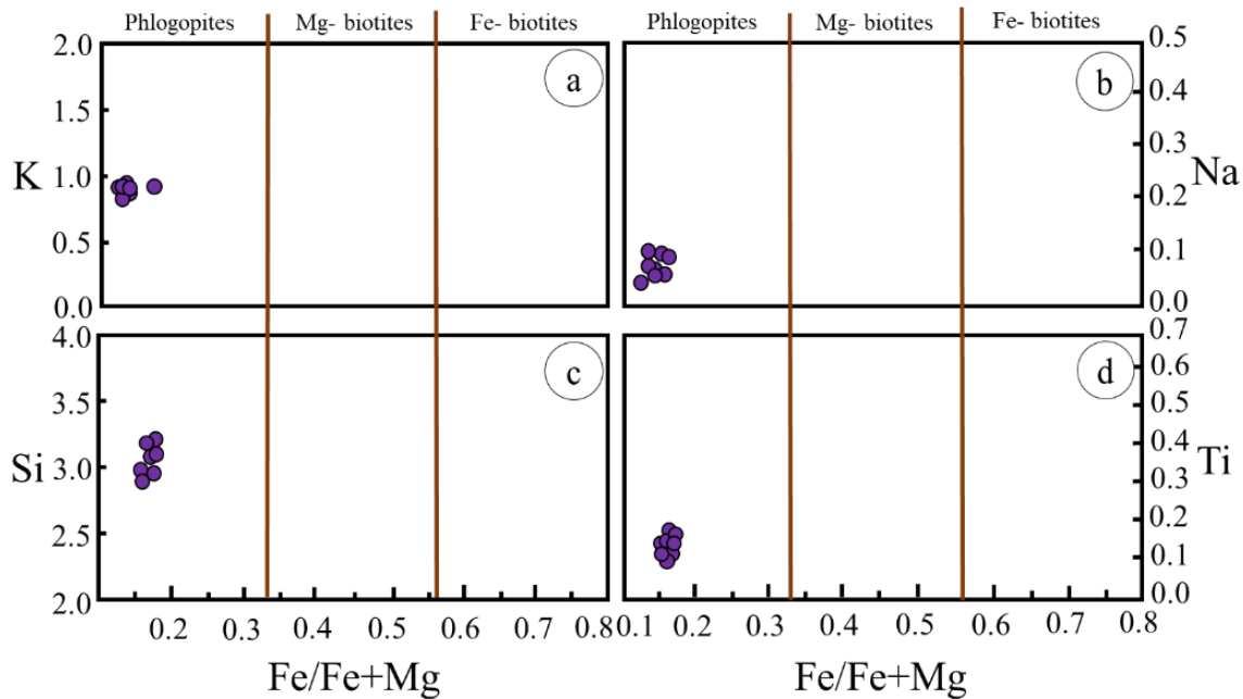
شکل ۱۸- ترکیب میکاهای مورد مطالعه بر روی نمودار تغییرات فراوانی برخی عناصر در برابر Fe/(Fe+Mg) .
