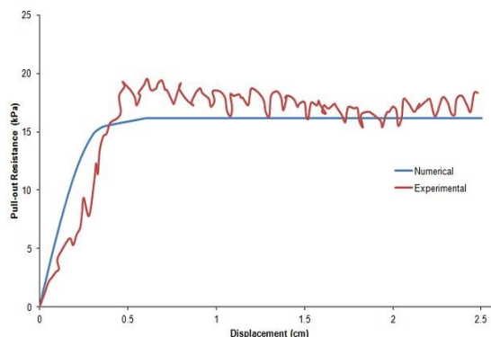
شکل ۱۴- تغییرات مقاومت در برابر تغییرمکان میخ A5 Fig. 14. Changes in strength to nail displacement A5
