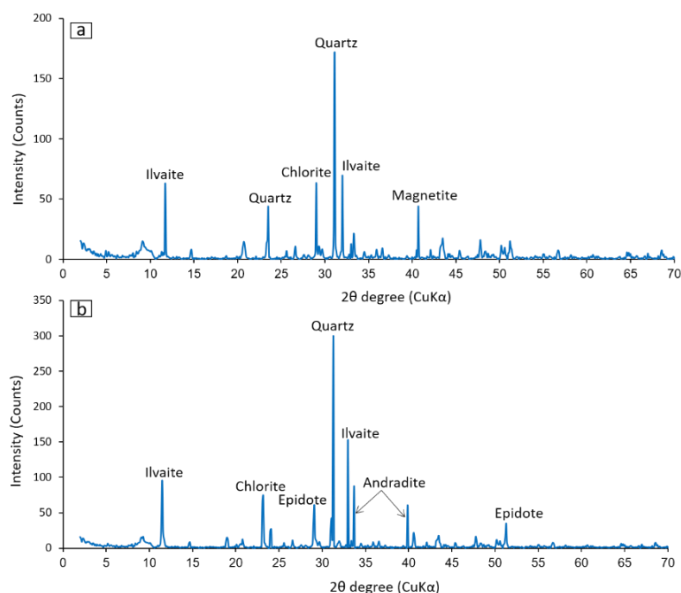
شکل ۵- تصاویر دیفرآکتوگرام XRD از بخش دگرسانی پسرونده و حضور ایلویت همراه کانی‌های دیگر.
