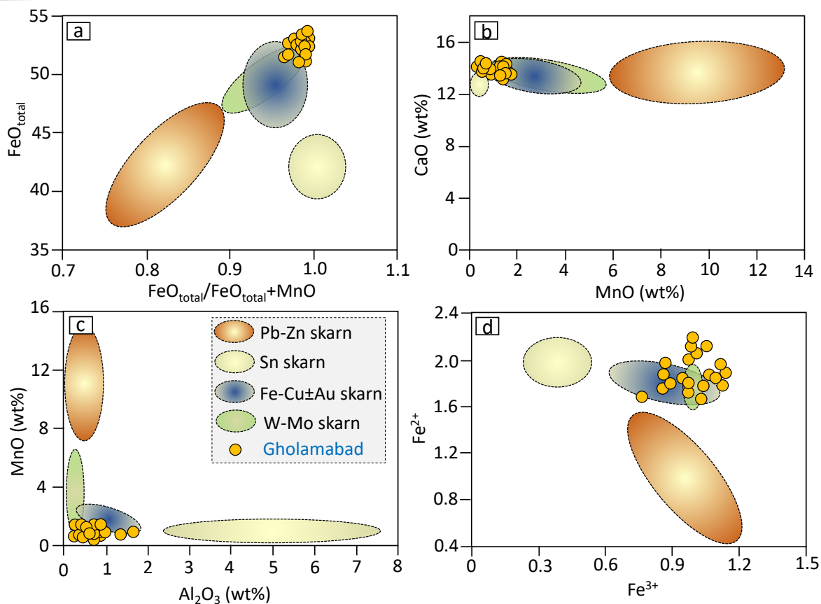
شکل ۹- نمودارهای دوتایی نسبت‌های مختلف عناصر اصلی برای ایلویت در کانسار آهن غلام‌آباد. (a) نمودار FeO_T در مقابل FeO / (FeO_T + MnO) نمودار. (b) نمودار CaO در مقابل MnO. (c) نمودار MnO در مقابل Al_2O_3 . (d) نمودار Fe^{2+} در مقابل Fe^{3+} . نمودار پایه از جیانگ و همکاران (Jiang et al., 2020).
