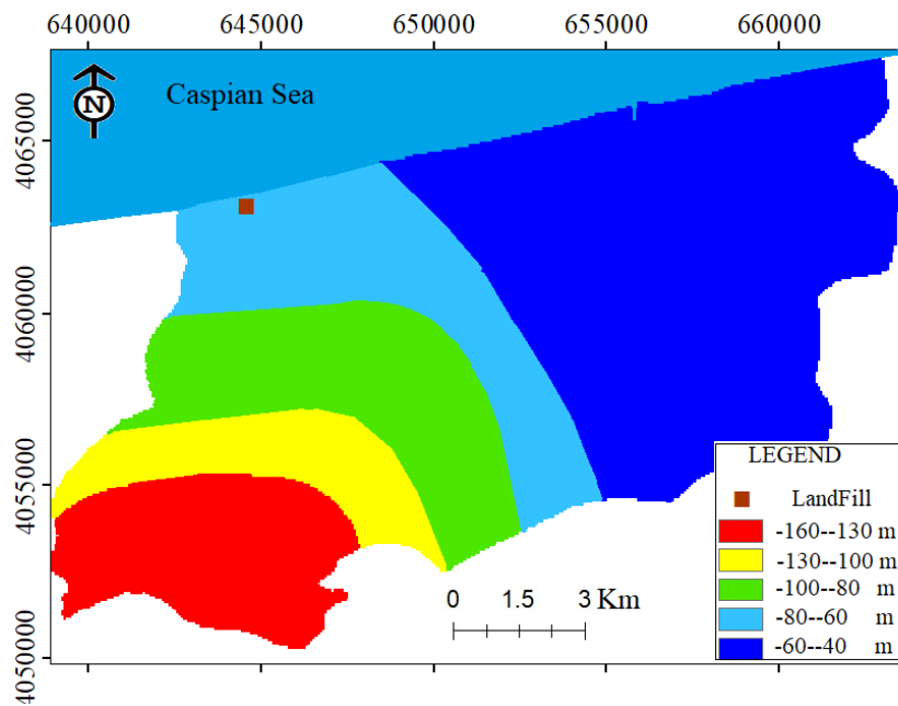
شکل ۴- نقشه سنگ کف آبخوان منطقه مورد مطالعه
