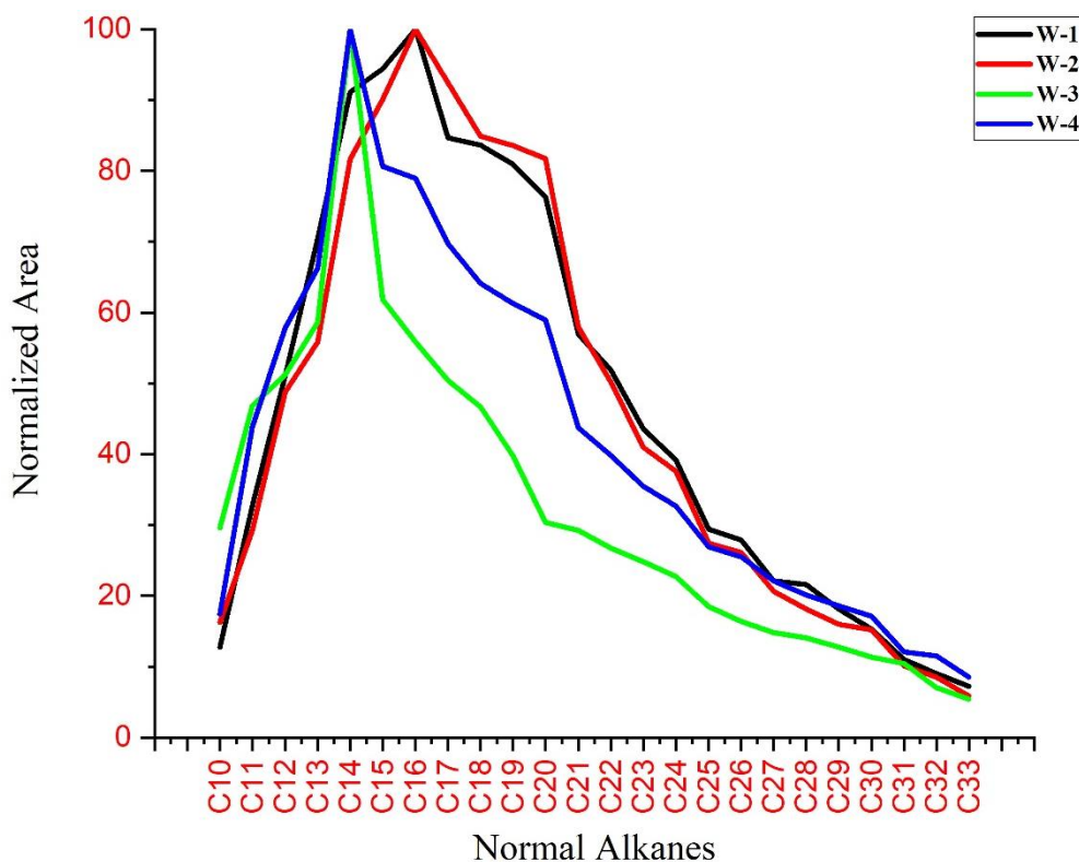
شکل ۶- توزیع نرمال آلکان‌ها در کروماتوگرام GC برای نمونه‌های مورد مطالعه.
