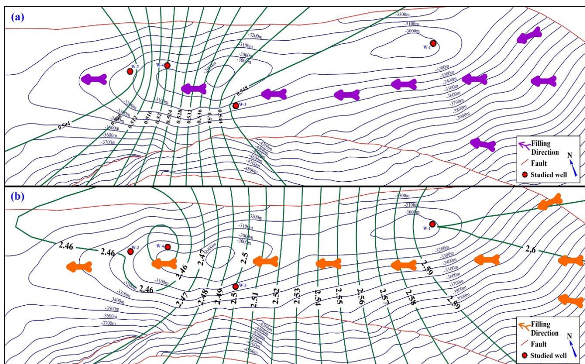
شکل ۸- نقشه‌های ایزوپلت برای (a) پارامتر غیر بایومارکری MDR، و (b) پارامتر بایومارکری \alpha\beta/(\alpha\alpha+\alpha\beta) C29 برای نمونه‌های مورد مطالعه.
