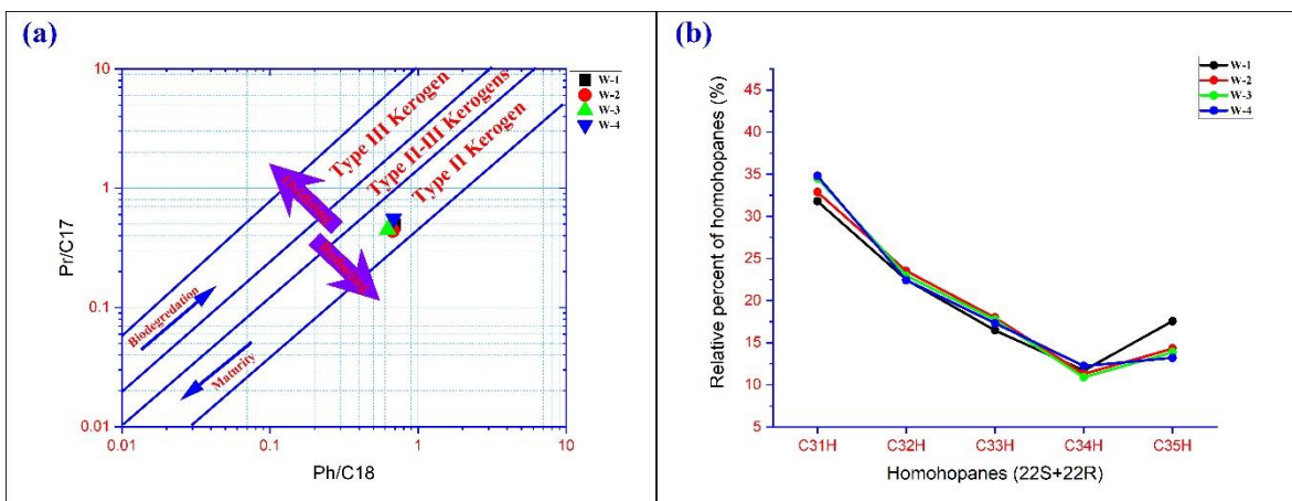
شکل ۵- (a) نمودار Ph/C18 در مقابل Pr/C17؛ (b) توزیع فراوانی همولوگ های هموئوپان ها (Peters et al., 2005). Fig. 5. a) Plot of Pr/C17 vs. Ph/C18; b) Distribution of different homologs of homohopanes (Peters et al., 2005).
