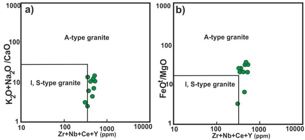
شکل ۸- نمودارهای متمایز کننده گرانیت‌های نوع A از گرانیت‌های نوع I و S (Whalen et al., 1987). نمودار (a) Zr+Ce+Y+Nb در برابر نسبت (Na_2O+K_2O)/CaO . نمودار (b) Zr+Ce+Y+Nb در برابر نسبت FeO^1/MgO . A-type= Anorogenic type, I and S type= Igneous and Sedimentary types
