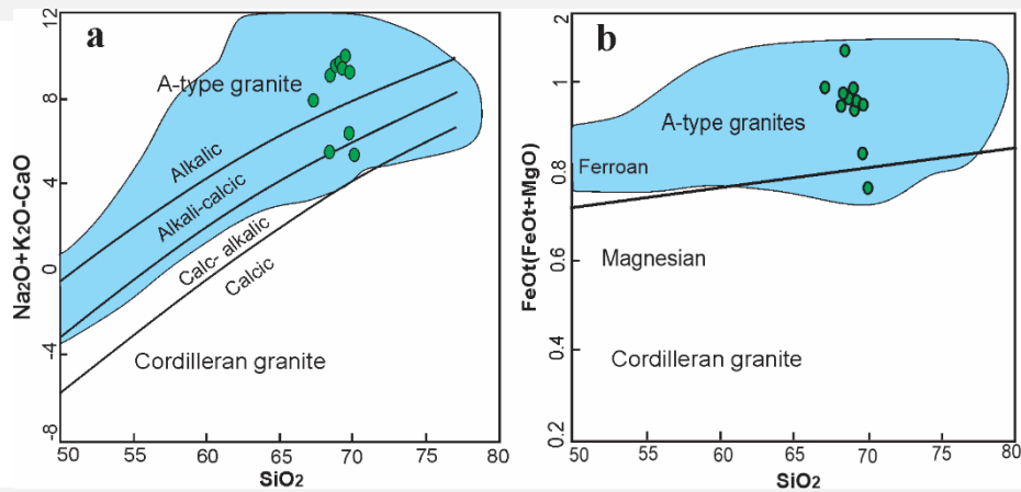
شکل ۹- نمودار (a) Na_2O+K_2O-CaO در مقابل SiO_2 (Frost et al., 2001). نمودار (b) نسبت FeO^1/(FeO^1 + MgO) در مقابل SiO_2 (Frost et al., 2001). محدوده آبی رنگ معرف دامنه ترکیب شیمیایی گرانیت‌های نوع A است (Vander Auwera et al., 2003).
