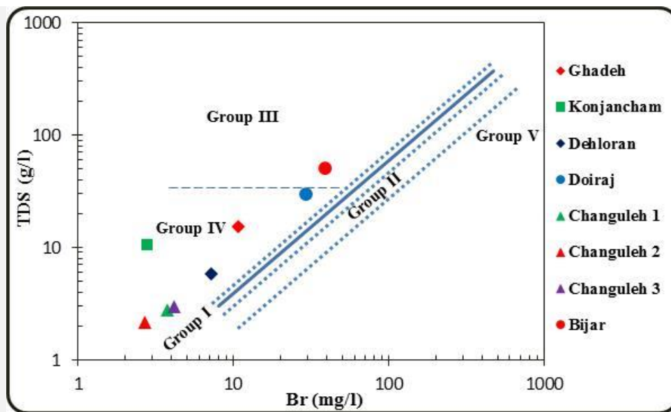
شکل ۹. نمودار رابطه TDS به Br چشمه‌های آبگرم و گوگردی استان ایلام
