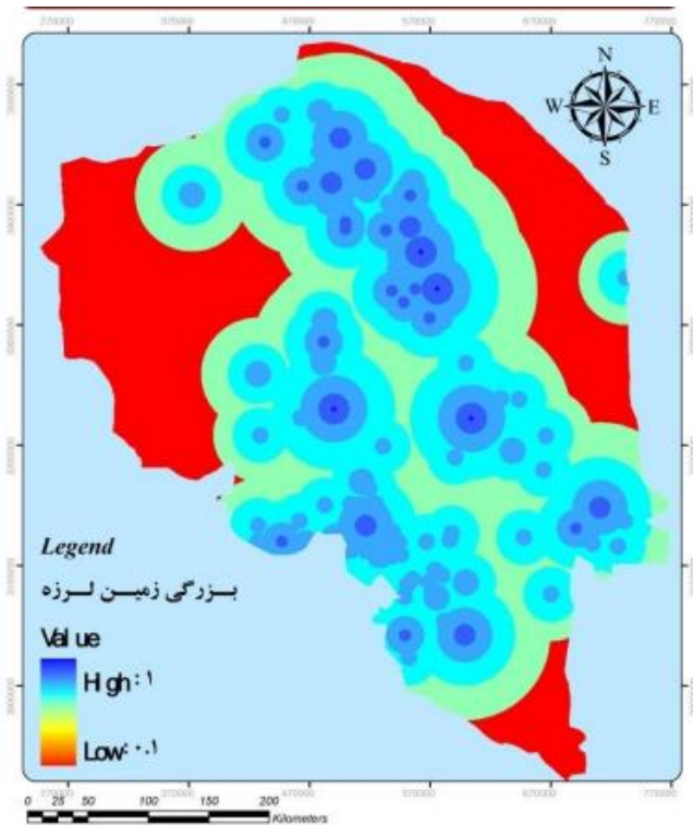
نگاره ۴- زیرمعیار بزرگای زمین لرزه‌ها. به دلیل پراکندگی روکانون زمین لرزه‌ها، نقشه یکنواختی خود را از دست داده است.
