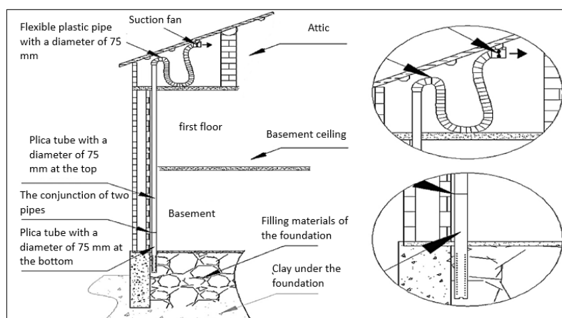
شکل ۳: طرح شماتیک اتخاذ روش دفع رادون با روش فن کشنده در یک واحد مسکونی Figure 2 Schematic plan of adopting the Radon disposal suction fan method in a residential unit
