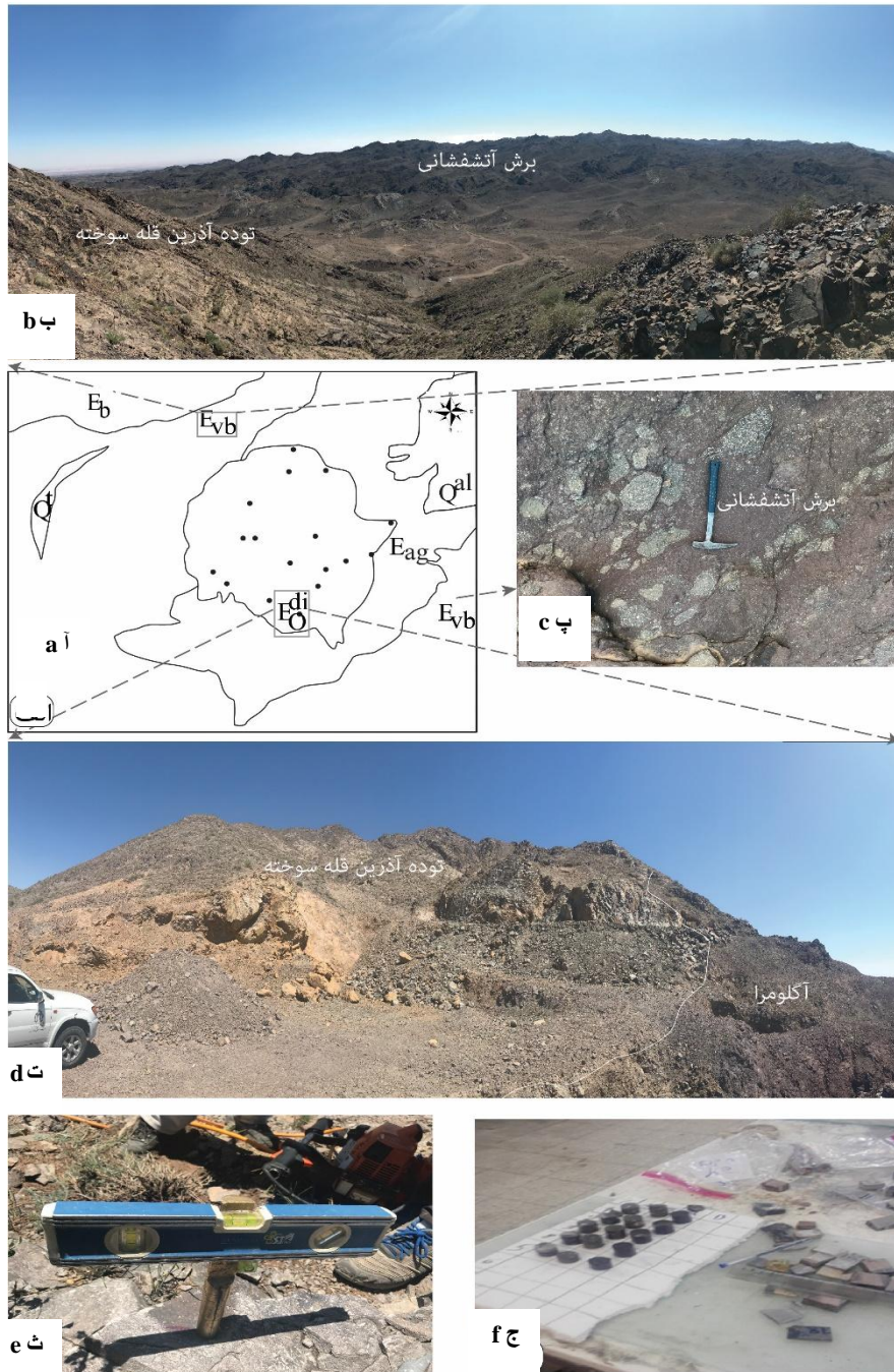
شکل ۲. آ) نقشه زمین‌شناسی شماتیک محدوده بررسی شده، ب) دورنمایی از واحدهای آتشفشانی-آذرآواری ائوسن در حاشیه شمال باختر توده قله سوخته (دید به سمت باختر)، پ) تصویر صحرایی از برش‌های آتشفشانی، ت) دورنمایی از توده نیمه-عمیق بررسی شده و سنگ‌های میزبان آن (دید به سمت شمال)، ث) برداشت مغزه‌های جهت‌دار به منظور بررسی‌های فابریک
