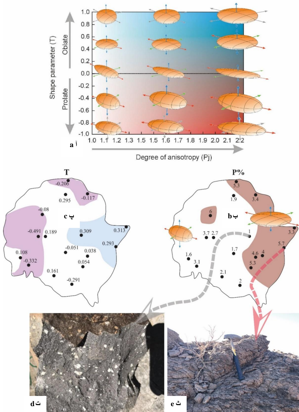
شکل ۶. آ) نمودار درجه ناهمسانگردی در مقابل پارامتر شکل (Mamtani et al., 2012)، ب) نقشه درصد ناهمسانگردی (P%) در توده قله سوخته. ایستگاه‌های با ناهمسانگردی بالا و پایین به ترتیب با رنگ‌های صورتی و خاکستری نشان داده شده است، پ) نقشه فاکتور شکل بیضوی مغناطیسی (T) که در آن ایستگاه‌های دارای بیضوهای مغناطیسی پهن و کشیده به ترتیب با رنگ‌های آبی و صورتی از یکدیگر متمایز شده‌اند، ت) تصویر نمونه دستی از دیوریت پورفیری توده‌ای در ایستگاهی با P% پایین، ث) فرسایش پوست پیازی در حاشیه درونی توده قله سوخته در ایستگاهی با P% بالا.
