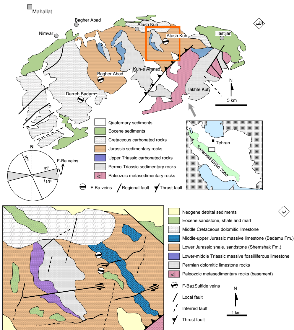
شکل ۱. الف) نقشه زمین شناسی منطقه جنوب شرق محلات واقع در بخش شمالی پهنه ساندج-سیرجان و موقعیت کانسارهای فلونوریت آتش کوه، دره بادام و باقرآباد در آن (با تغییرات از [۱۸]، ب) نقشه زمین شناسی ساده شده منطقه آتش کوه که در آن موقعیت و راستای رگه های فلونوریت-باریت-سولفید نمایش داده شده است
